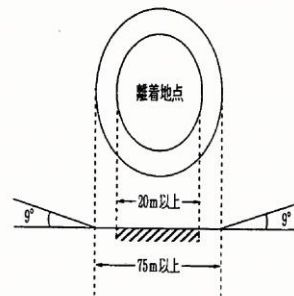
d 大型機 (CH-47, SH-60J) の場合
