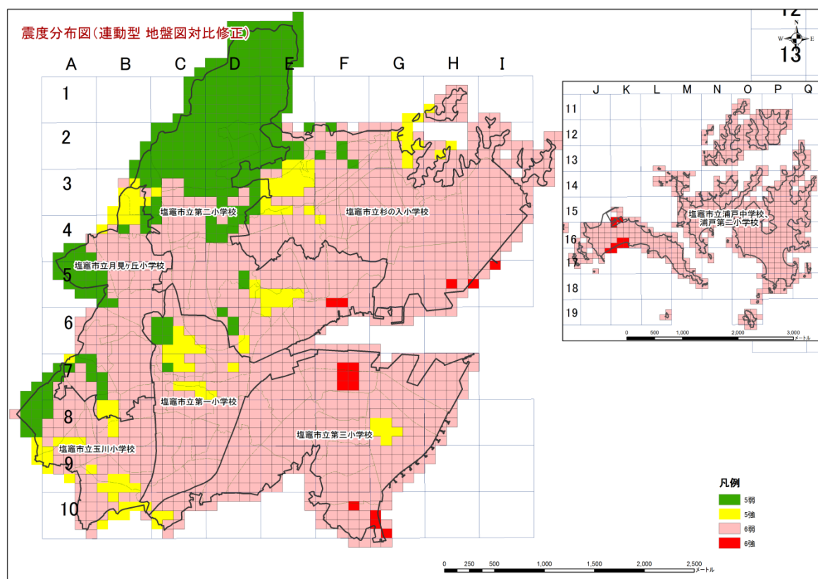
図1－4 塩竈市の震度分布図（宮城県沖地震連動型 Mw=8.0）
