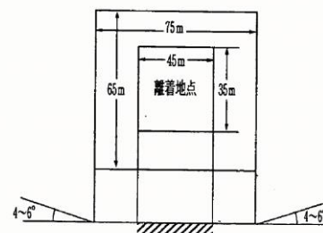
d 大型機 (CH-47, SH-60J) の場合
