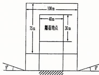
c 大型機 (V-107) の場合
