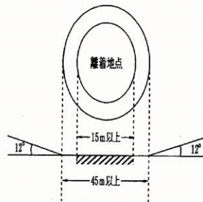
c 大型機 (V-107) の場合
