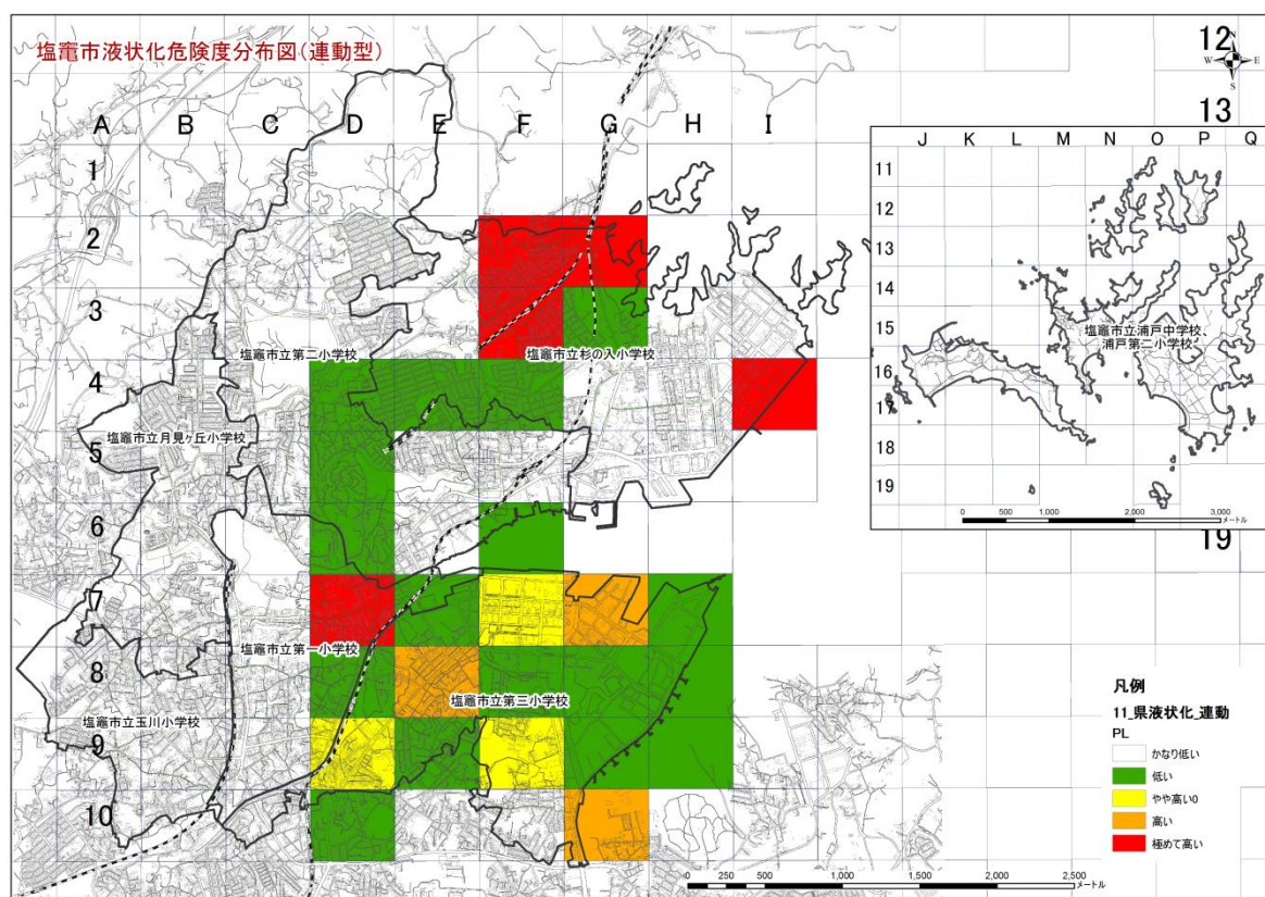
図1－5 塩竈市の液状化危険度（宮城県沖地震連動型 Mw=8.0）
